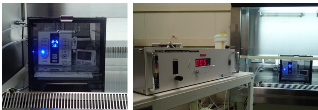
本研究における試験の様子。左：デシケーター内でのオゾン曝露の様子。右：オゾン濃度モニターによるオゾン濃度の制御。
