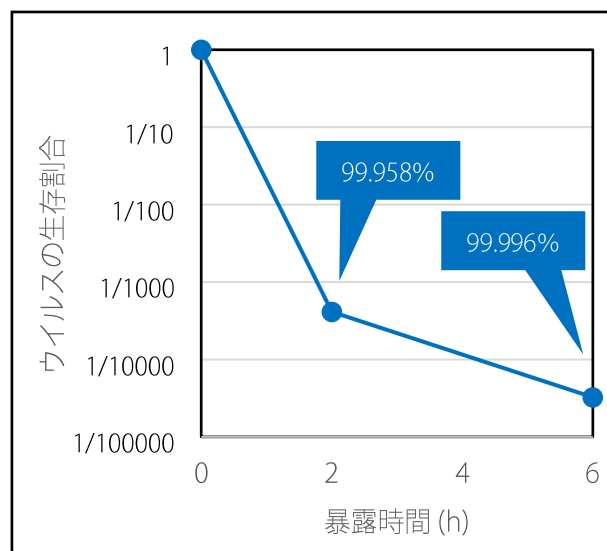
図2：オゾンによるウイルスの生存割合
