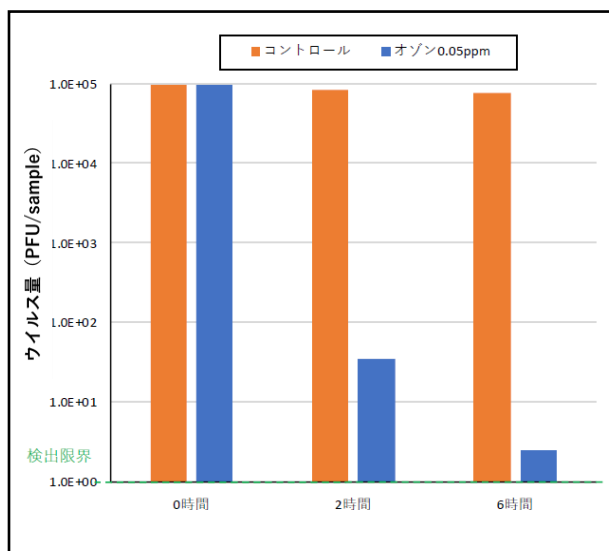
図1：オゾンによるウイルス量の変化
